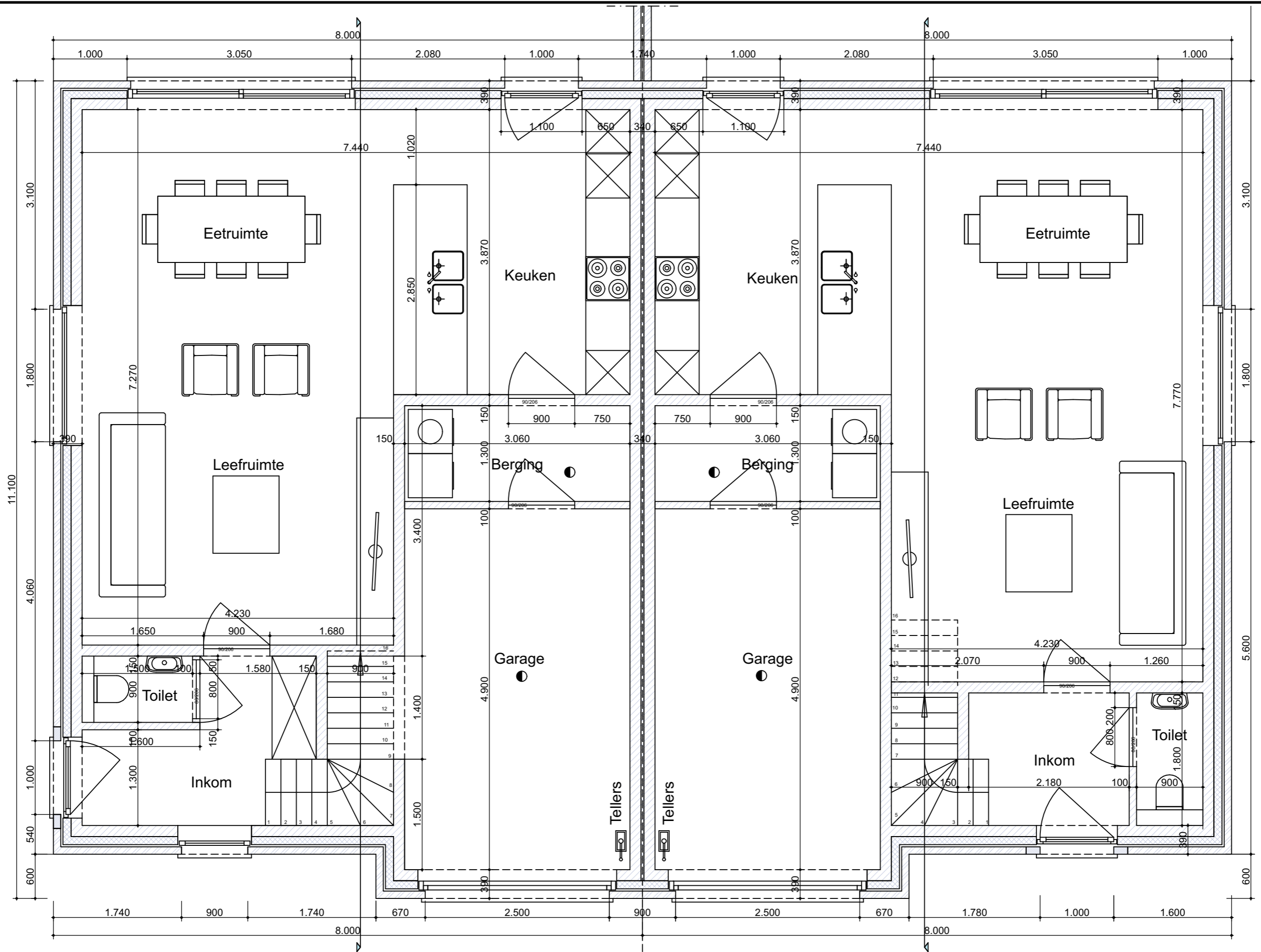
Grondplan
